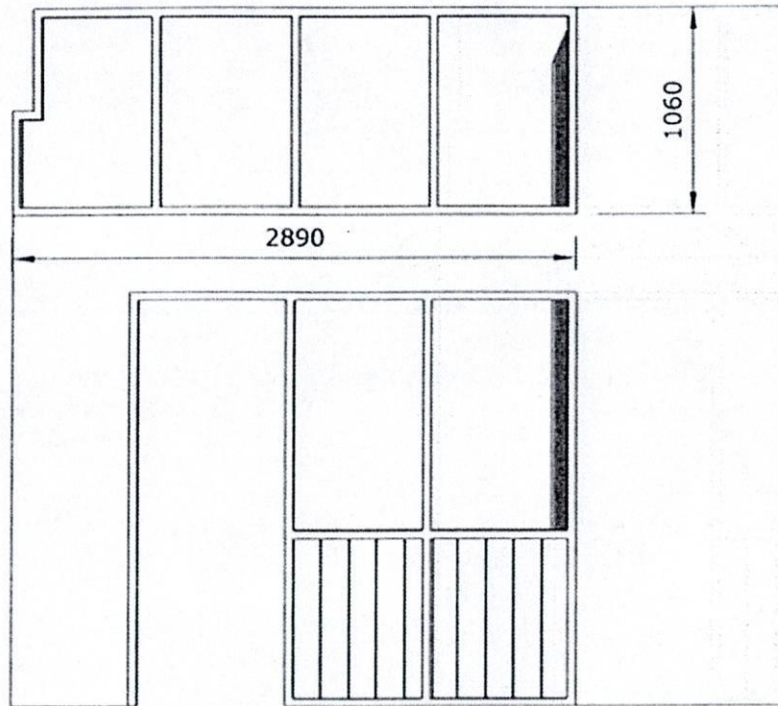
MẶT DỰNG
