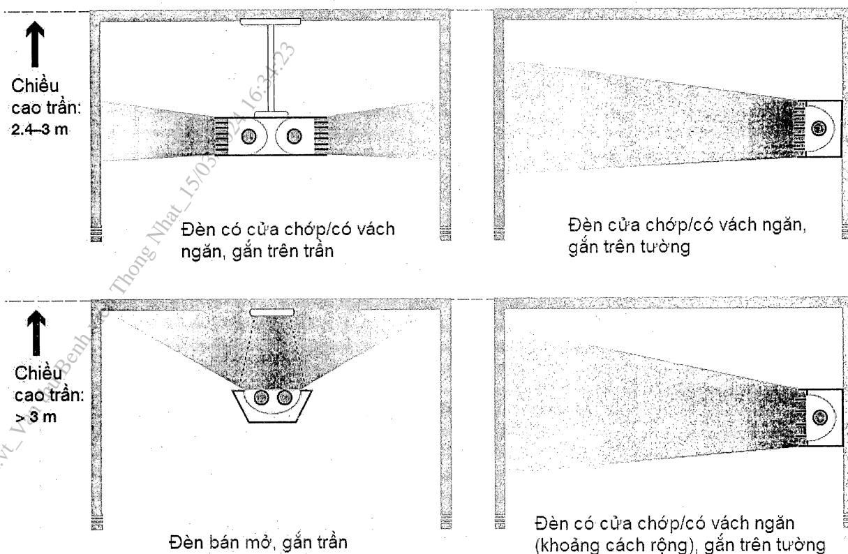
Hình 8: Các loại đèn GUV tăng trần phù hợp với chiều cao phòng khác nhau 20
