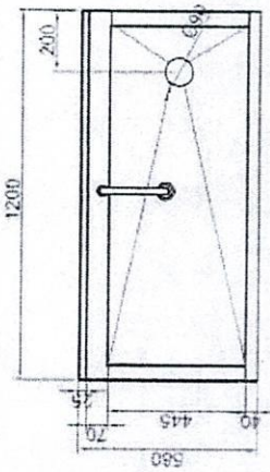
FRONT VIEW Scale: 1:1
